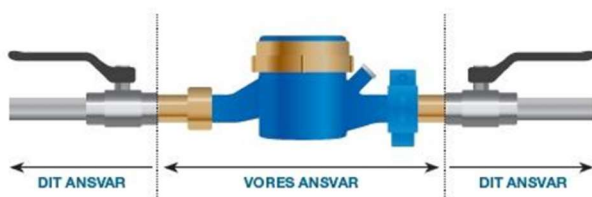
Ansvarsfordeling i vandinstallationen
